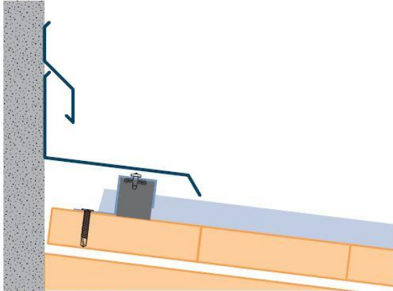
Falstage contre mur
