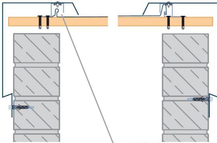
Rive tombante de fin sur mur
