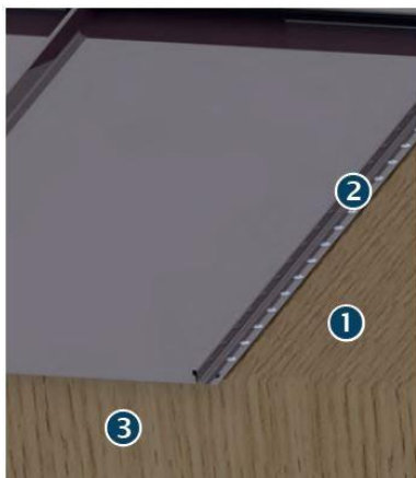
1. Voliges épaisseur 15 mm minimale 2. Perforation par pas de 50 mm 3. Bandeau
