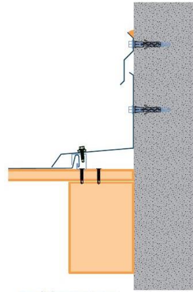
Rive de depart contre mur
